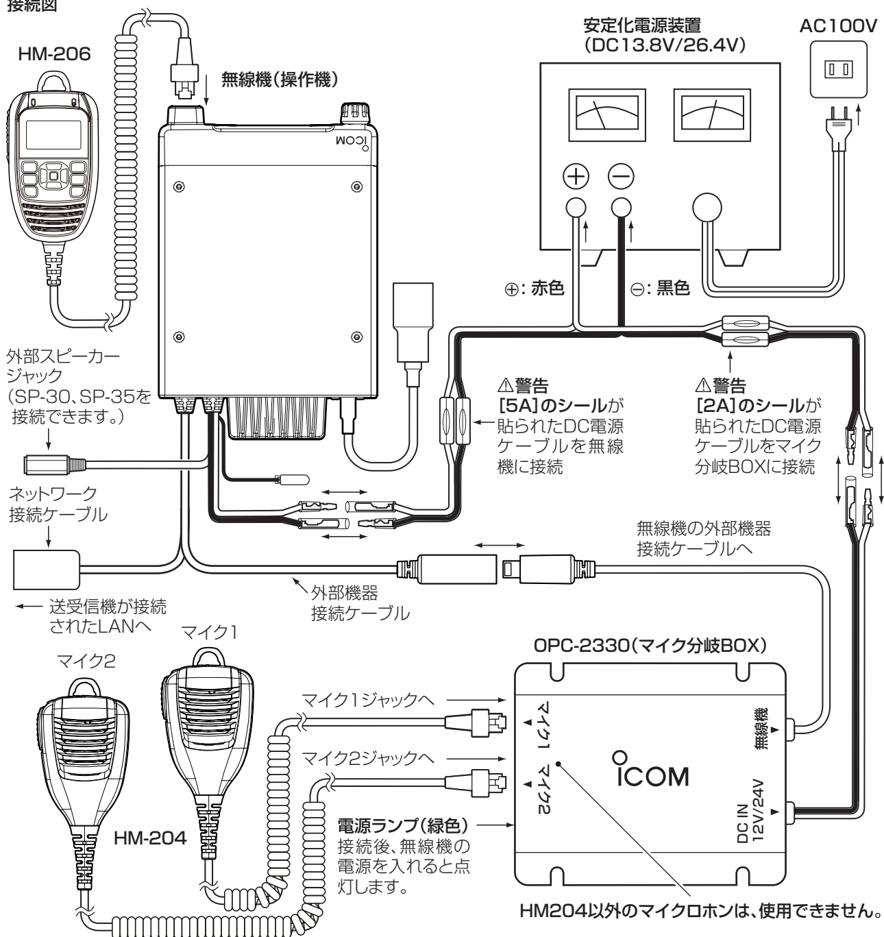
接続図
